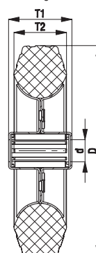
Rollenlager
